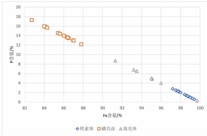
图一三 东平陵硅钙系炉渣铁颗粒各金相组织 P-Fe 含量分布图
