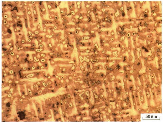
图一四 铜刻刀89T7⑦: 11的金相组织(α树枝晶铸造组织, 夹杂少量的铜硫化物和砷化物颗粒)
