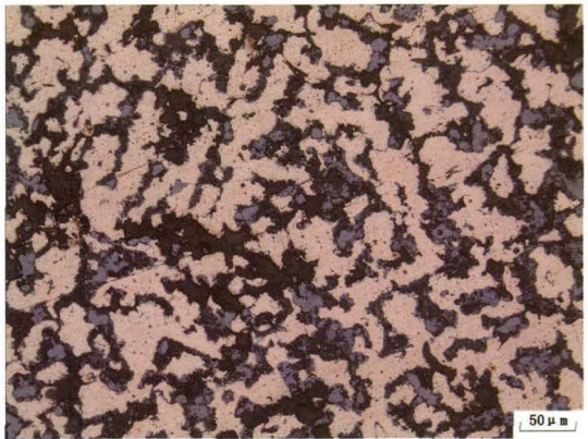
图一五 残铜器10TCST8⑦: 4的金相组织(α固溶体树枝晶偏析, 灰色岛屿状相为γ相)
