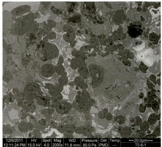
图七 师姑墩炉壁挂渣T5⑥：1背散射电子像 (三种相均为铅青铜)
