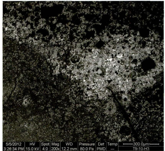
图六 师姑墩炉壁T9H3：1背散射电子像（右侧部分为铜锈，亮白色为高铅锡相）
