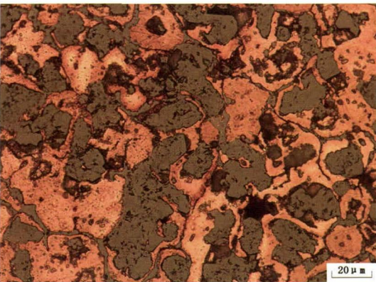
图一三 铜镞89T8⑥: 6的金相组织(α大晶粒, 灰色部分是腐蚀所致)
