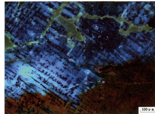
图一六 铜矛10TCST7③: 1暗场下显微组织(基本α树枝晶组织)
