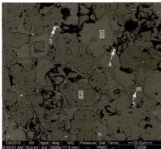
图一七 铜镞89T8⑥：6背散射电子像 (EDS微区分析：1. 铜基体 2. 锈蚀区 3~5. 夹杂物)
