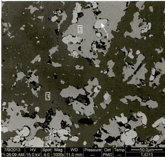
图四 汤家墩铜矿石T3⑧：1背散射电子像 (EDS微区分析：1. 重晶石 2. 硫化矿相 3. 氧化矿相)
