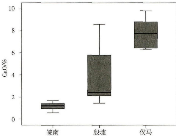
图九 陶范样品CaO含量的箱式图
