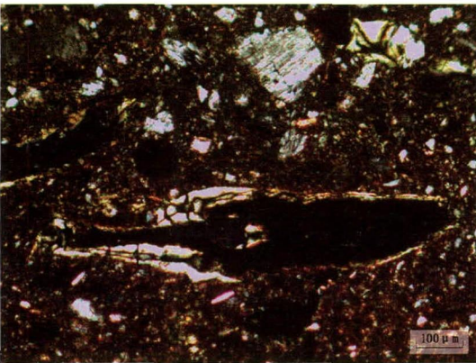
图一二 陶范89T6⑥: 8显微组织夹杂的炭化稻壳
