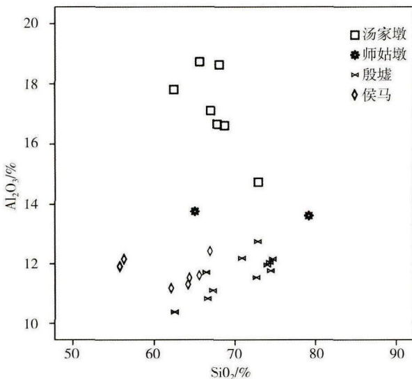
图一〇 陶范样品Si-Al二维因子散点图
