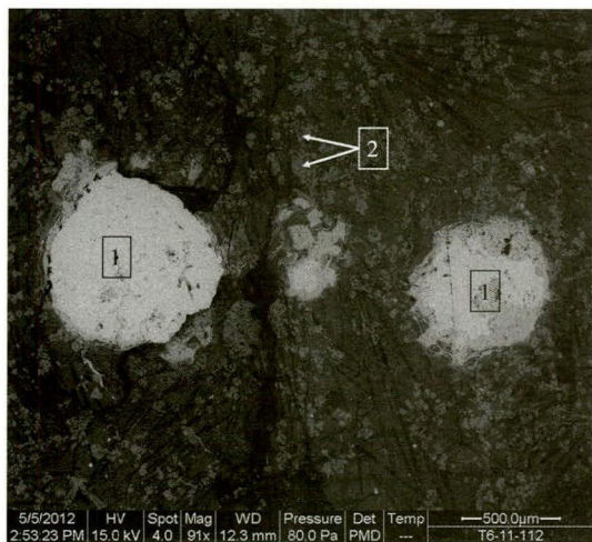
图二 师姑墩炉渣10TCST6：112背散射电子像 （EDS微区分析：1. 红铜颗粒 2. 浮氏体）
