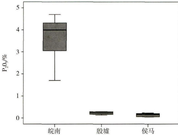
图八 陶范样品P 2 O 5 含量的箱式图
