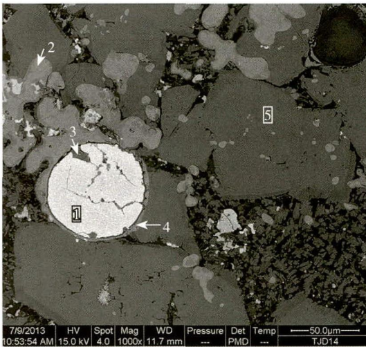
图五 汤家墩炉渣T3⑧:2背散射电子像 (EDS微区分析：1. 冰铜颗粒 2、4. 铁氧化物 3. 铜铁砷相 5. 铁橄榄石)
