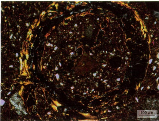
图一一 陶范89T7⑤: 1显微组织夹杂的炭化植物茎杆
