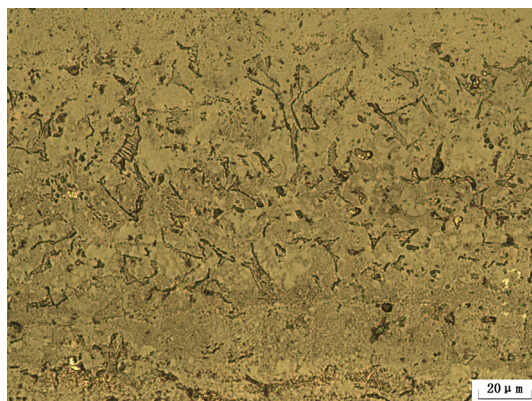
图六 残铁块 83042 锈蚀中铁素体+珠光体组织痕迹
