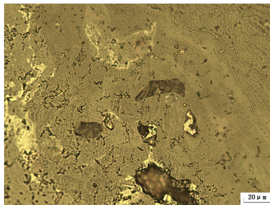
图二 残铁块 83035 锈蚀中的共晶夹杂物
