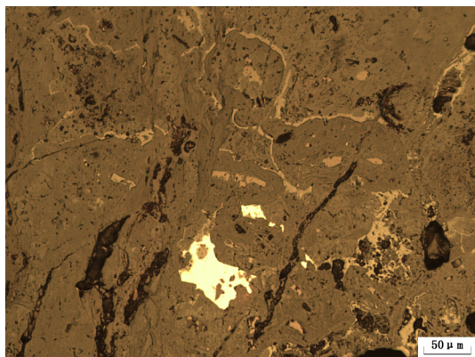
图三 残铁块 83035 锈蚀中的铁素体组织痕迹
