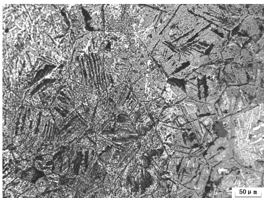
图五 残铁块 83039 锈蚀中的碳化析出物痕迹
