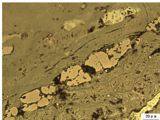
图四 残铁块 83037 锈蚀中的共晶夹杂物
