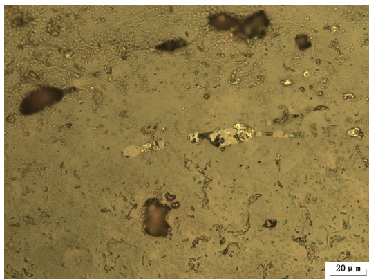
图一 残铁块 83034 锈蚀中的共晶夹杂物
